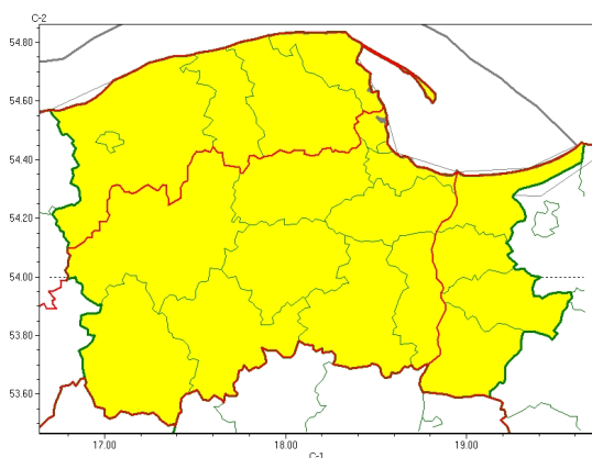
Oblodzenie 2025-01-02 21:35
