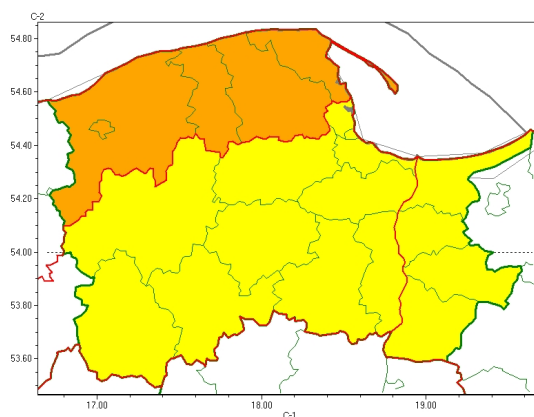
Silny wiatr 2025-01-02 21:35
